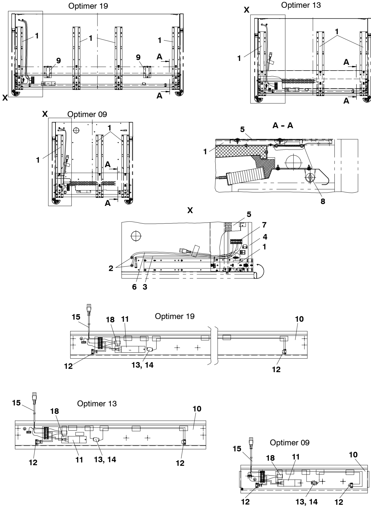
Fig. 8: Beleuchtung horizontal
