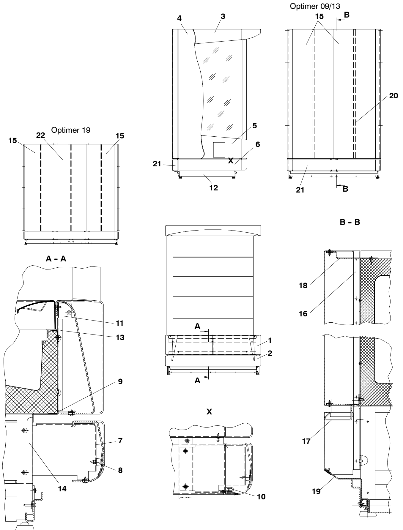
Fig. 2: Außenverkleidung und Rückwand
