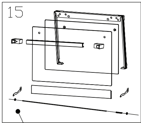
15 Door assembly
