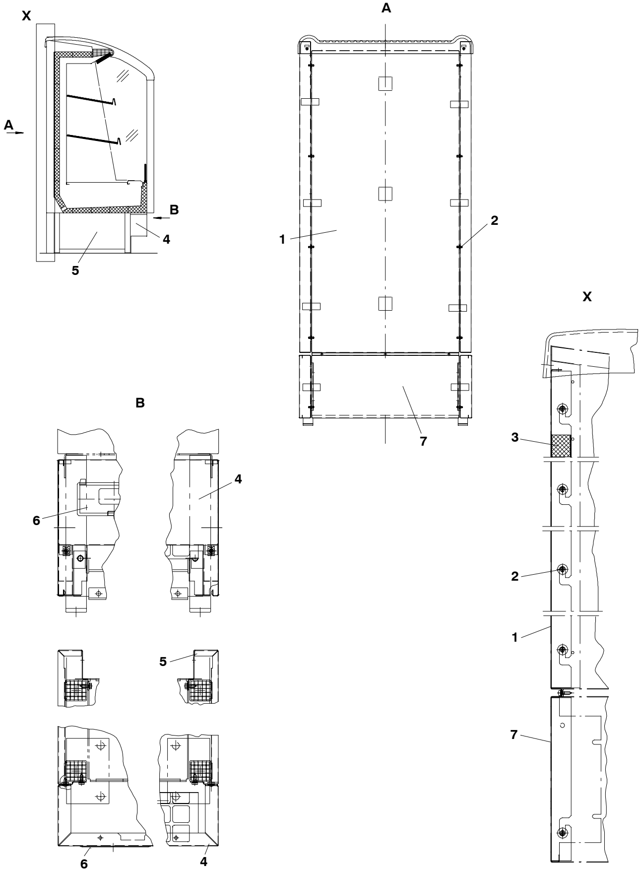
Fig. 2: Rückwandverkleidung, Sockelverkleidung
