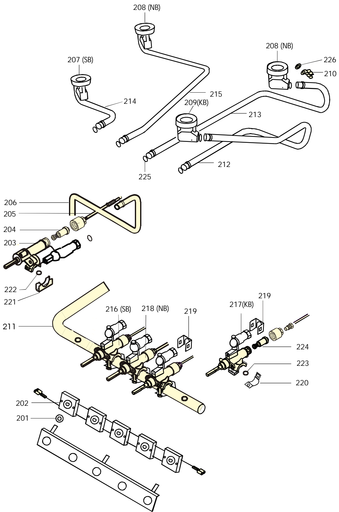
Hahngarnitur FGH60L2-4
