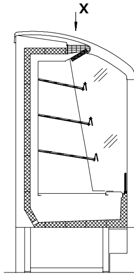
Fig. 3: Abdeckung
