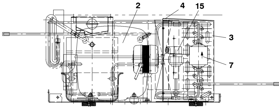
Fig. 11: Verflüssigungssatz
