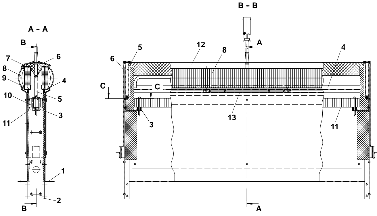
Fig. 6: Luftleitwand mitte NOPREMORWAN1
