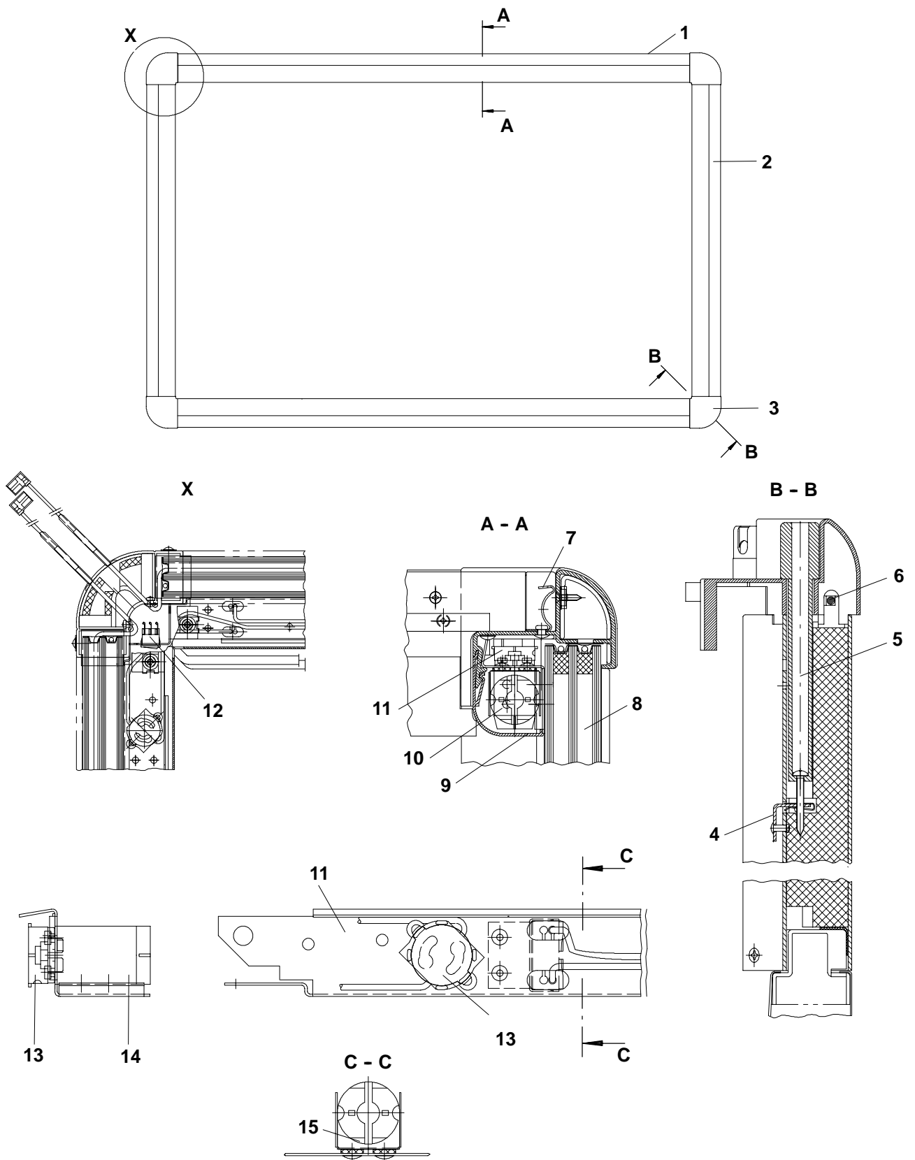
Fig. 2: Baugruppe Glasaufsatz mit Handlaufbeleuchtung N0PREMOROB1
