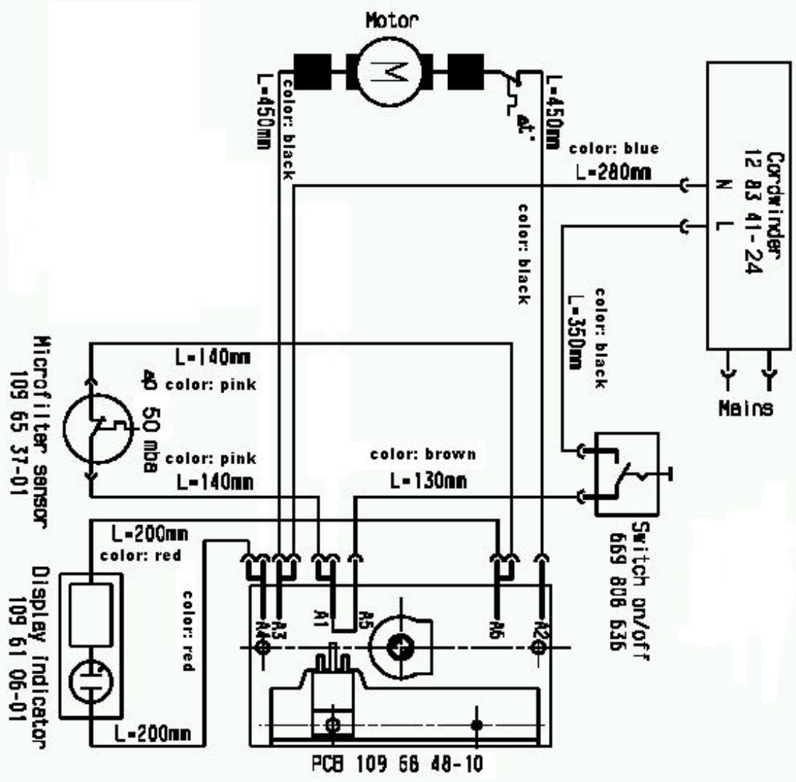
Wiring 109 68 83-10
