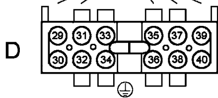
Ansicht: Bestückungsseite
