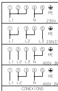
HOB SWITCH
