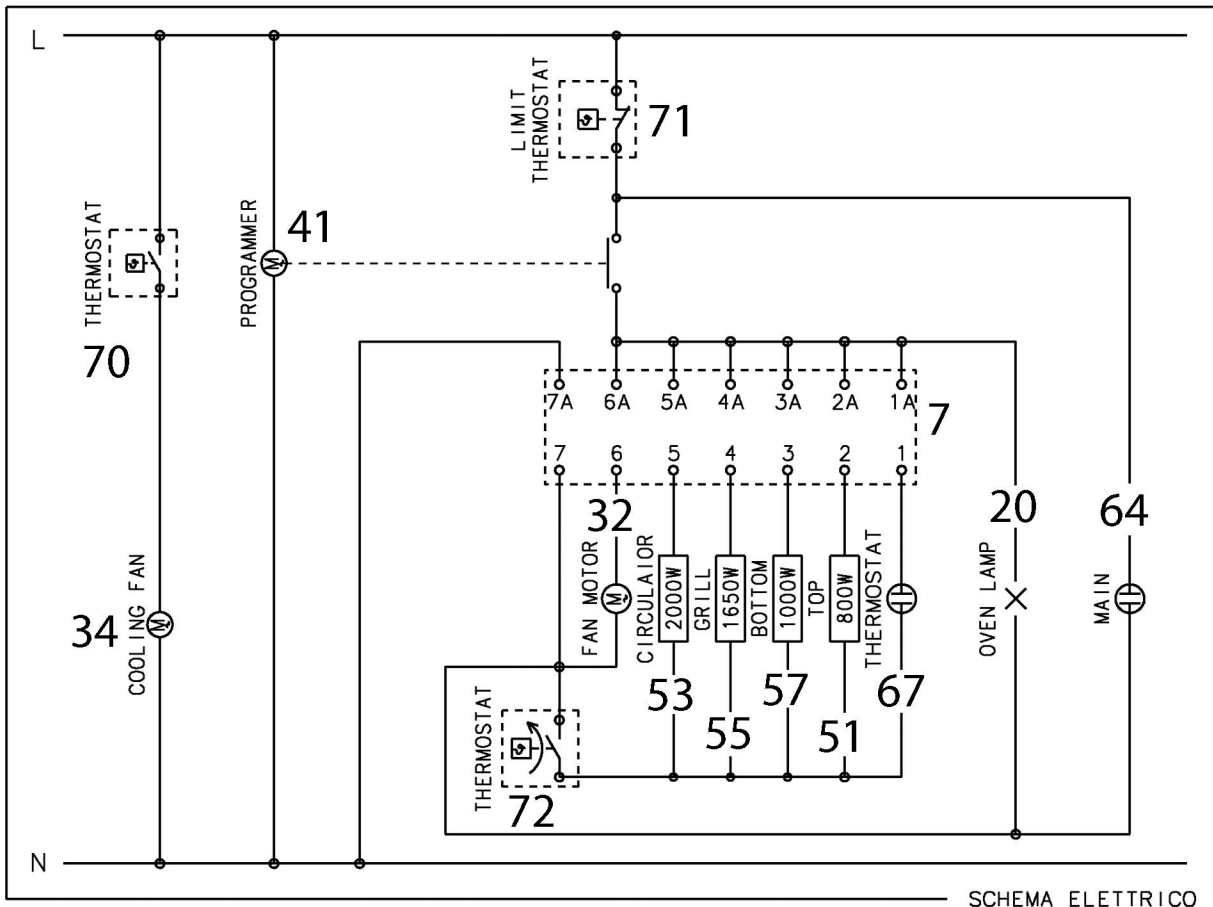
SCHEMA ELETTRICO
