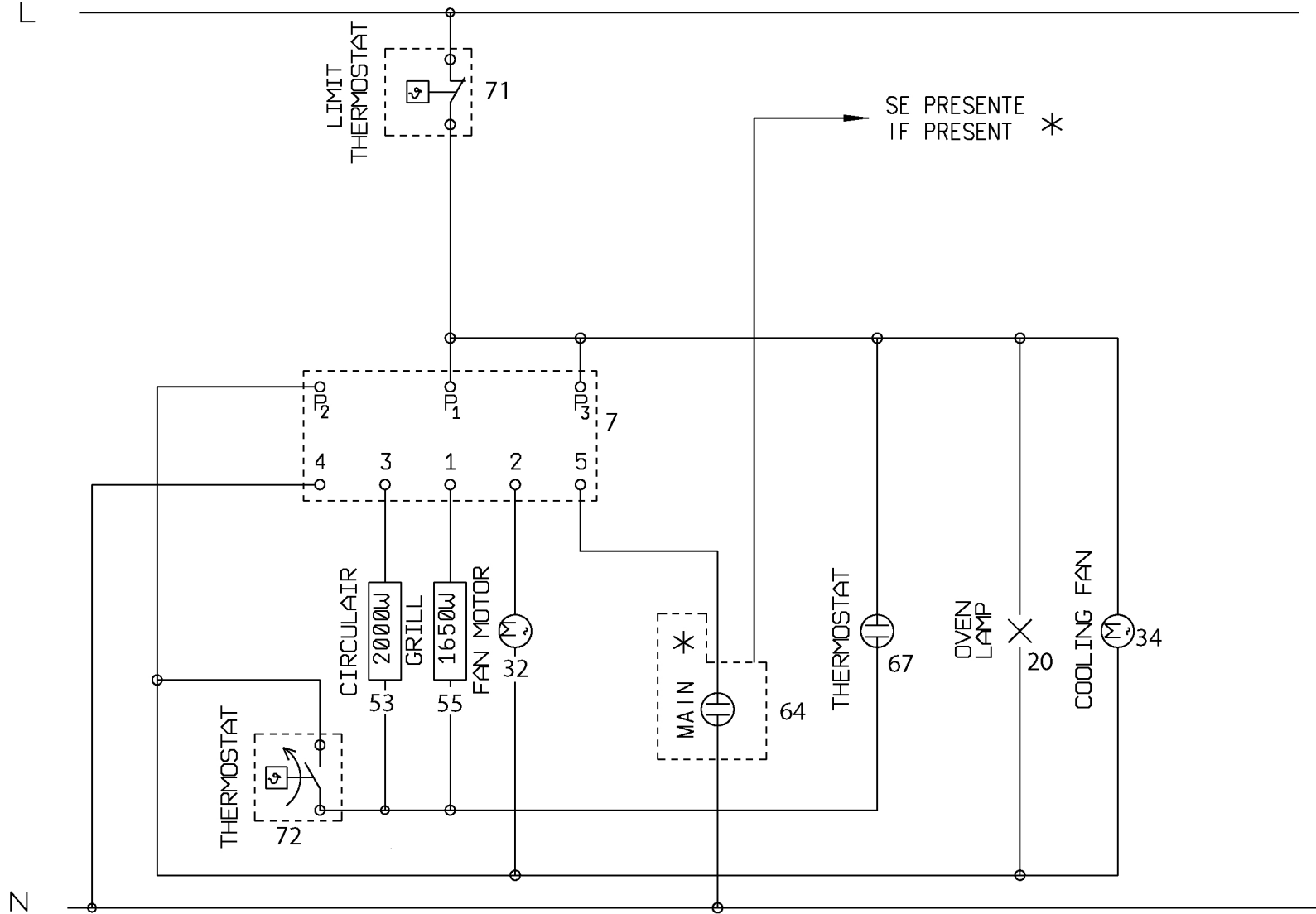
FUNCTIONAL DIAGRAM - SCHEMA FUNZIONALE
