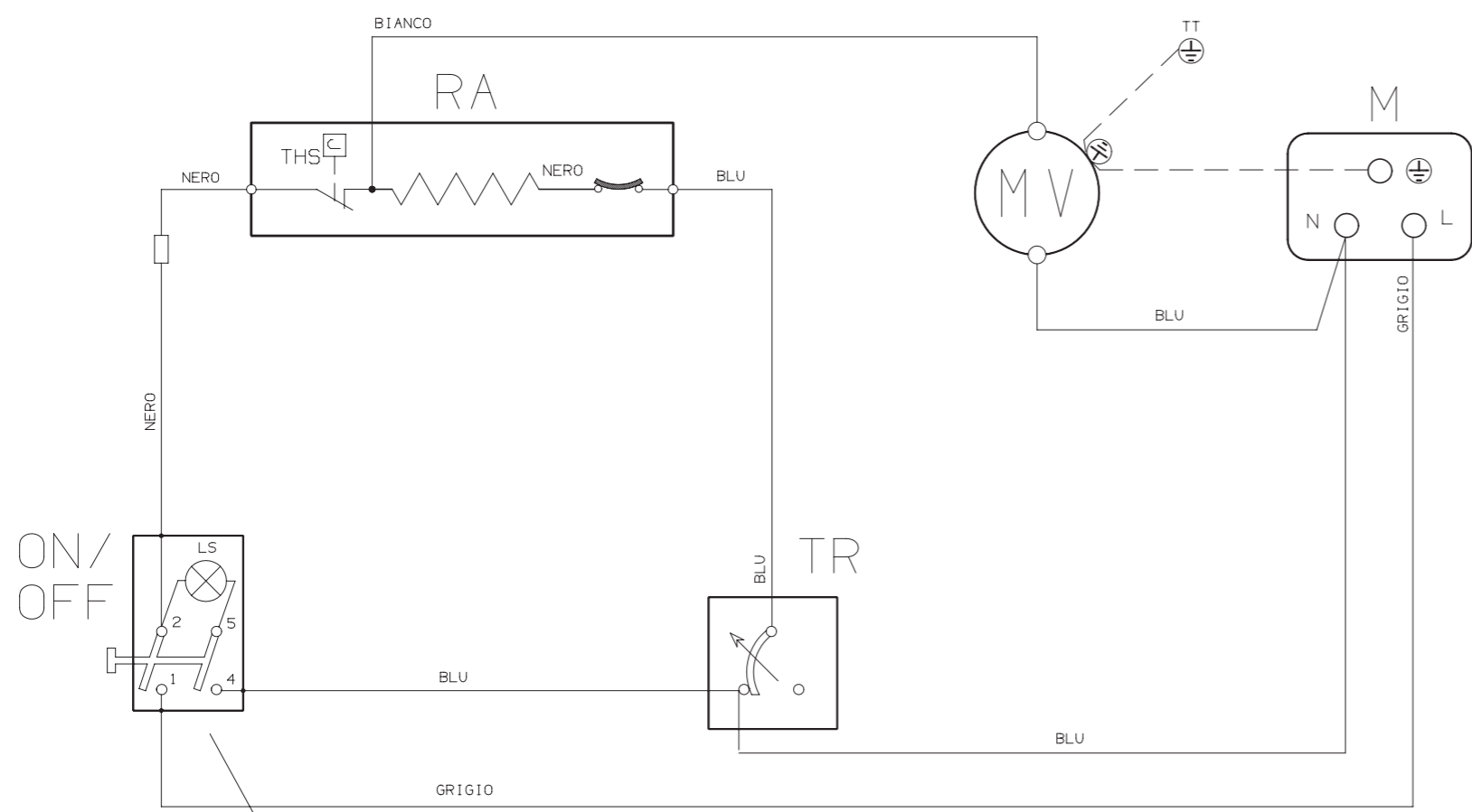
DETTAGLIO COLLEGAMENTI PULSANTE
