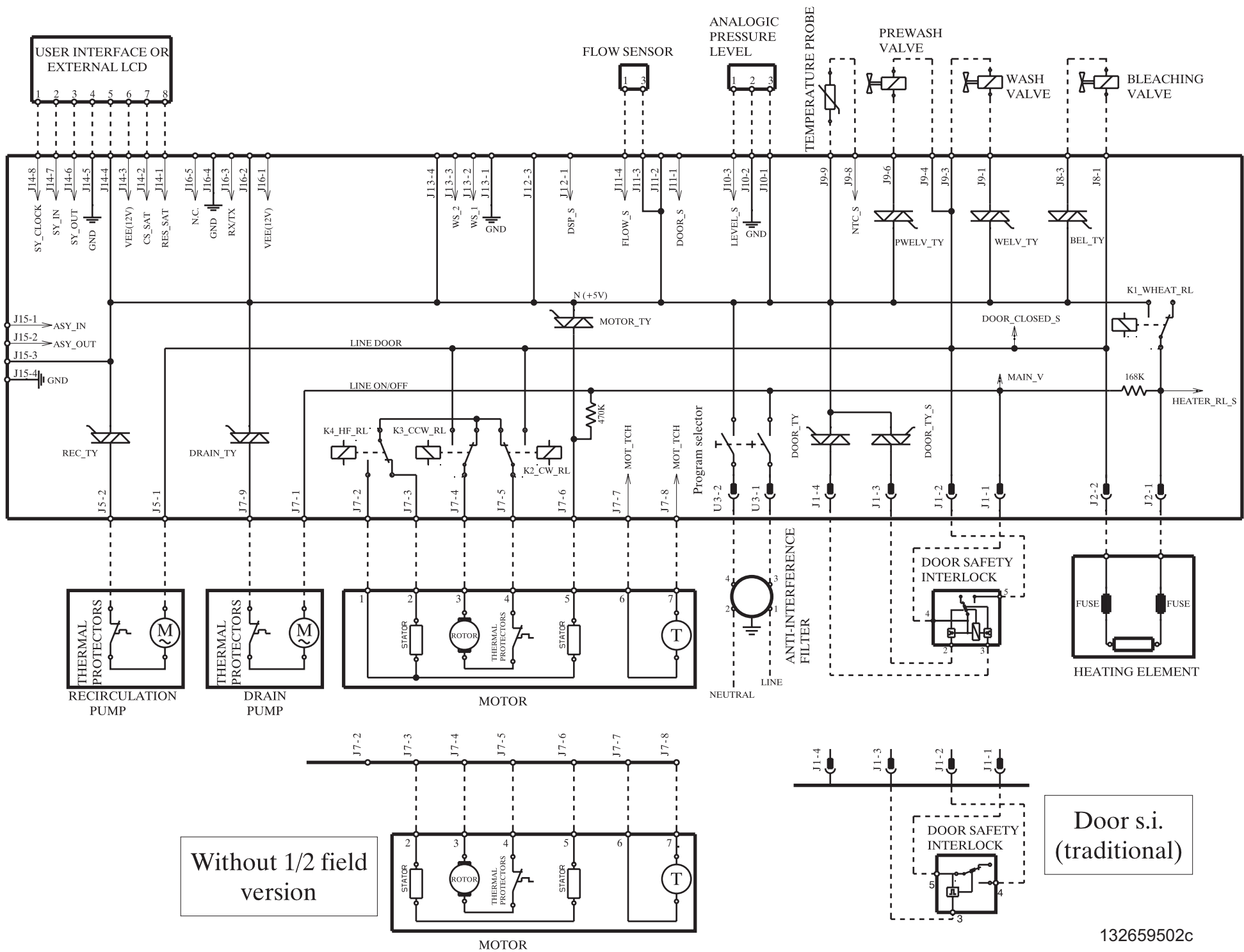
MOTOR
