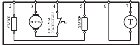
MOTOR
