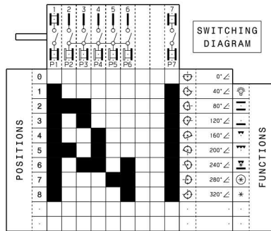
OVEN SWITCH 807180501
