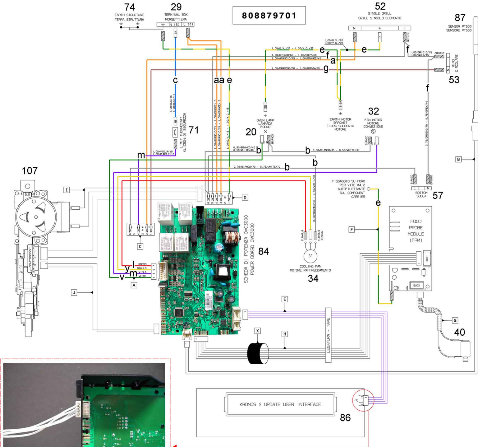
FIGURA DI ESEMPIO MONTAGGIO TASSATIVO COME DA FOTO (LA COLORAZIONE DEI CAVETTI RIPORTATI SULLA FOTO PUO ESSERE NON VERITIERA)
