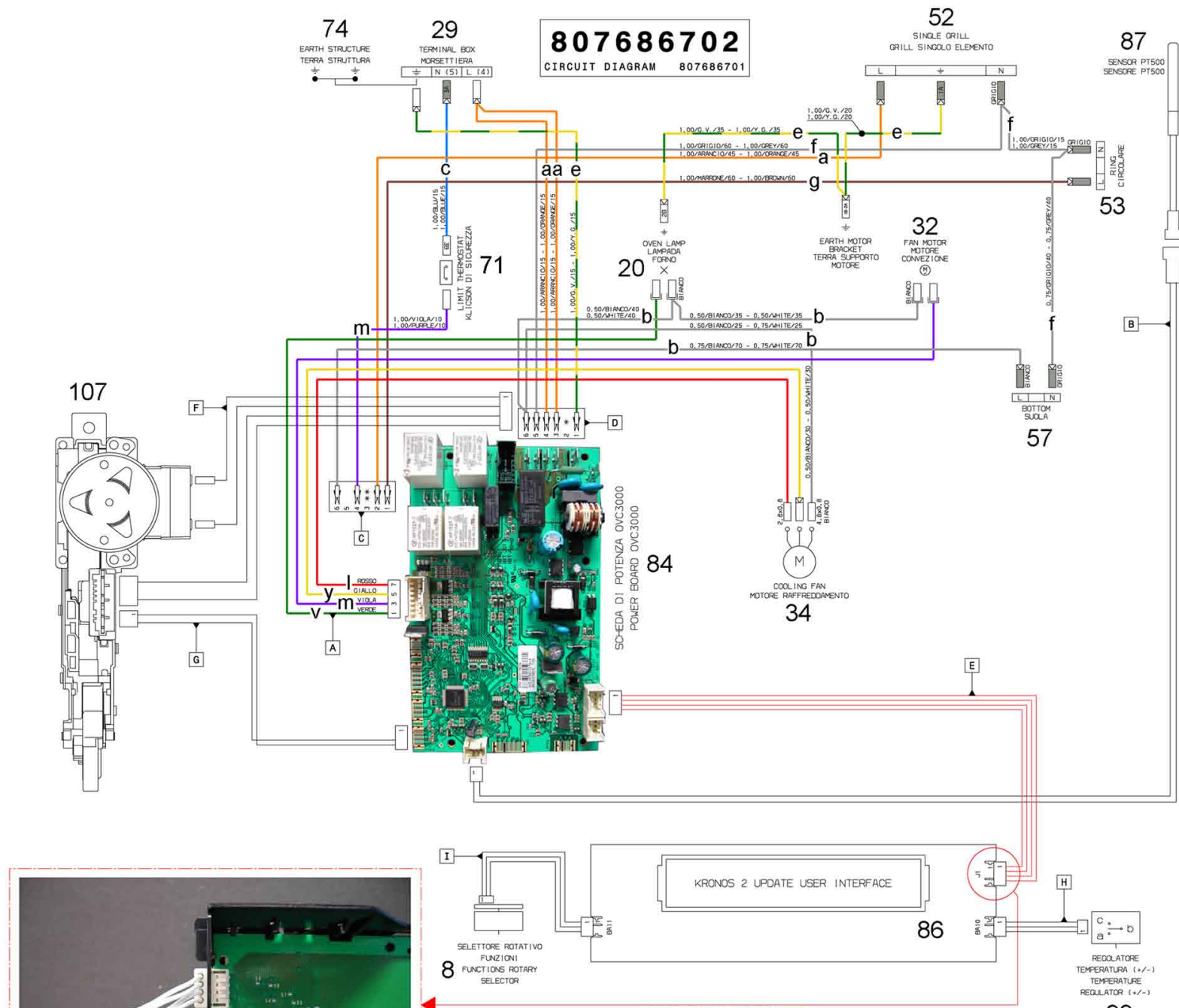
FIGURA DI ESEMPIO MONTAGGIO TASSATIVO COME DA FOTO (LA COLORAZIONE DEI CAVETTI RIPORTATI SULLA FOTO PUO ESSERE NON VERITIERA)
