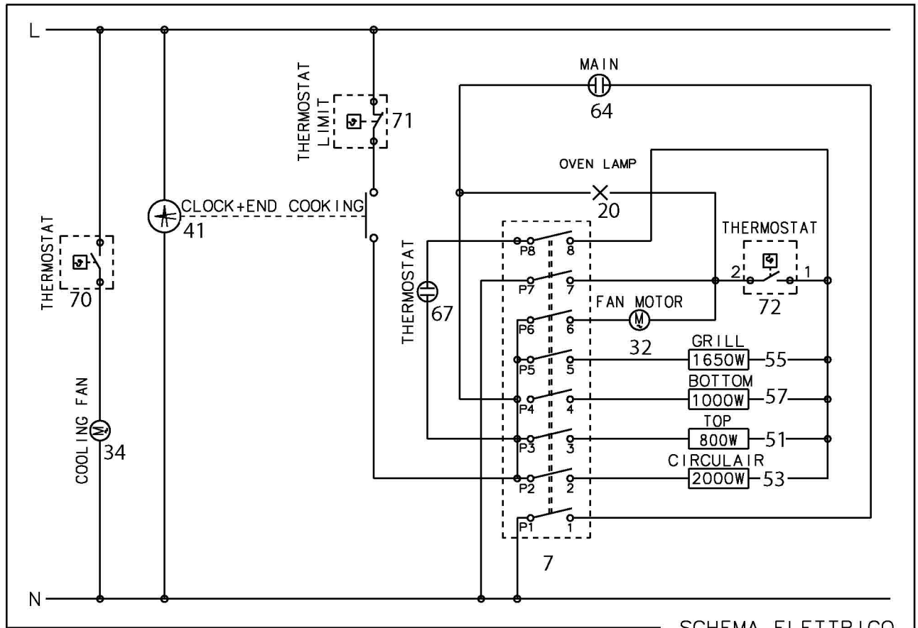
SCHEMA ELETTRICO
