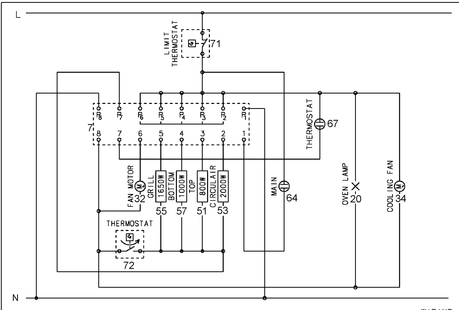
WIRING
