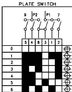
DISPOSIZIONE PIASTRE-FUOCHI
