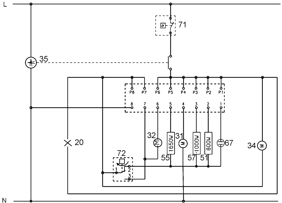
SCHEMA ELETTRICO
