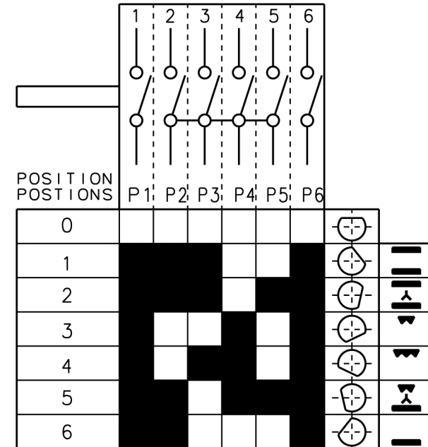
DIAGRAMMA ELETTRICO
