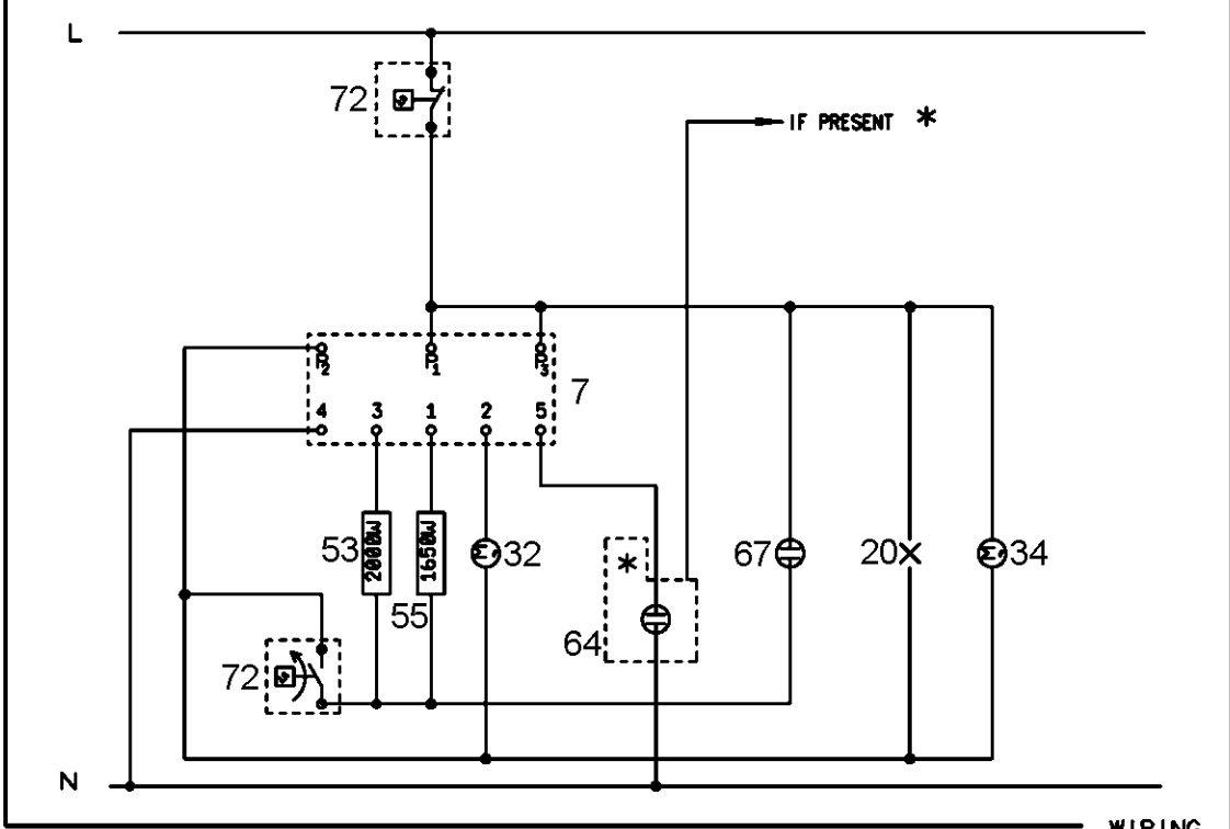
WIRING
