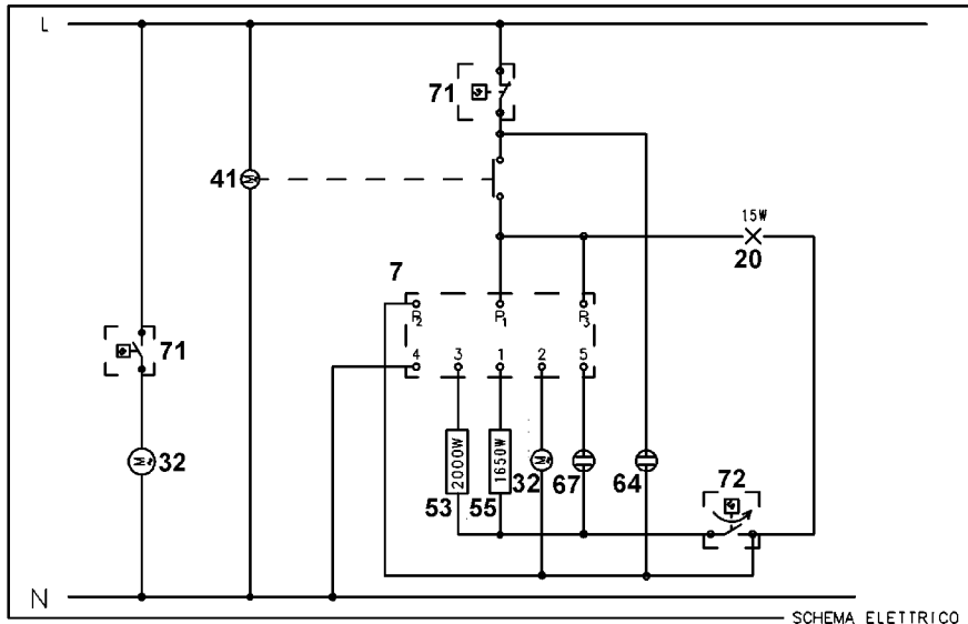
SCHEMA ELETTRICO
