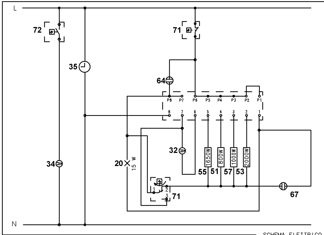
SCHEMA ELETTRICO
