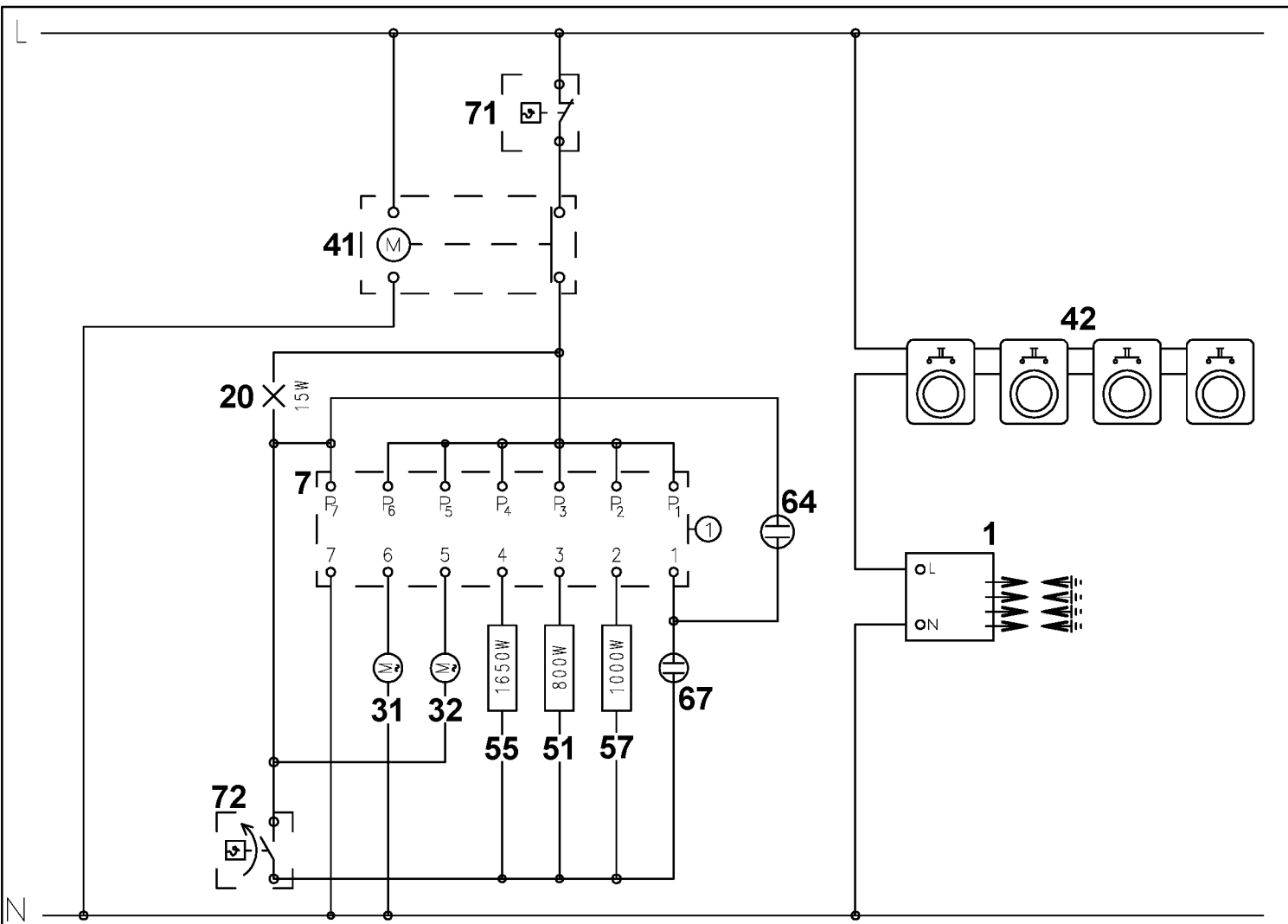
SCHEMA ELETTRICO
