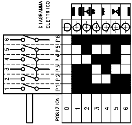
SCHEMA ELETTRICO
