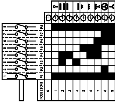
COLLEGAMENTI ELETTRICI
