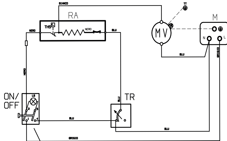
DETTAGLIO COLLEGAMENTI PULSANTE
