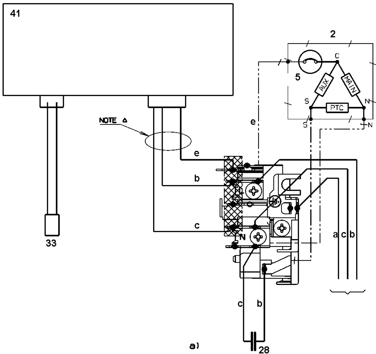
SCHEMA ELETTRICO "RAST 5"
