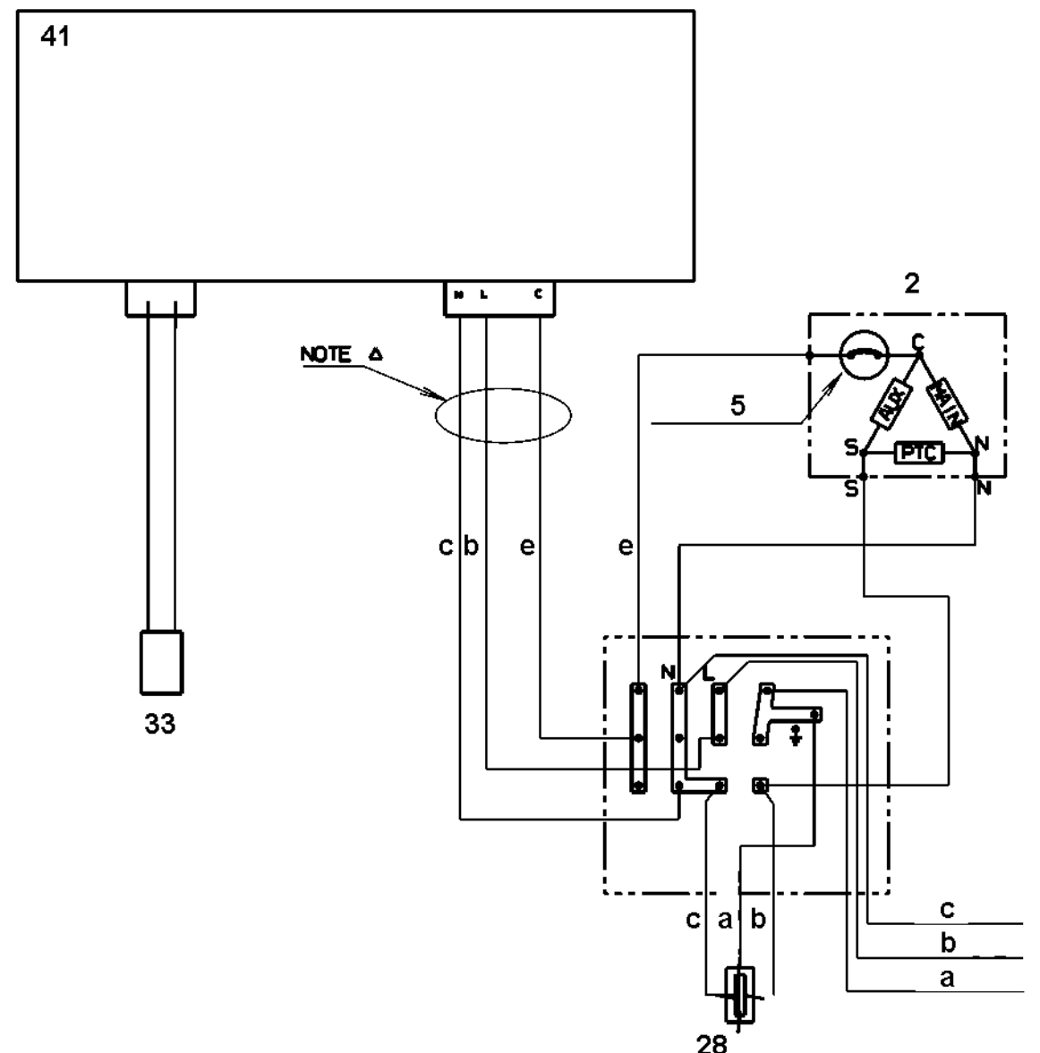
SCHEMA ELETTRICO "SET F2"
