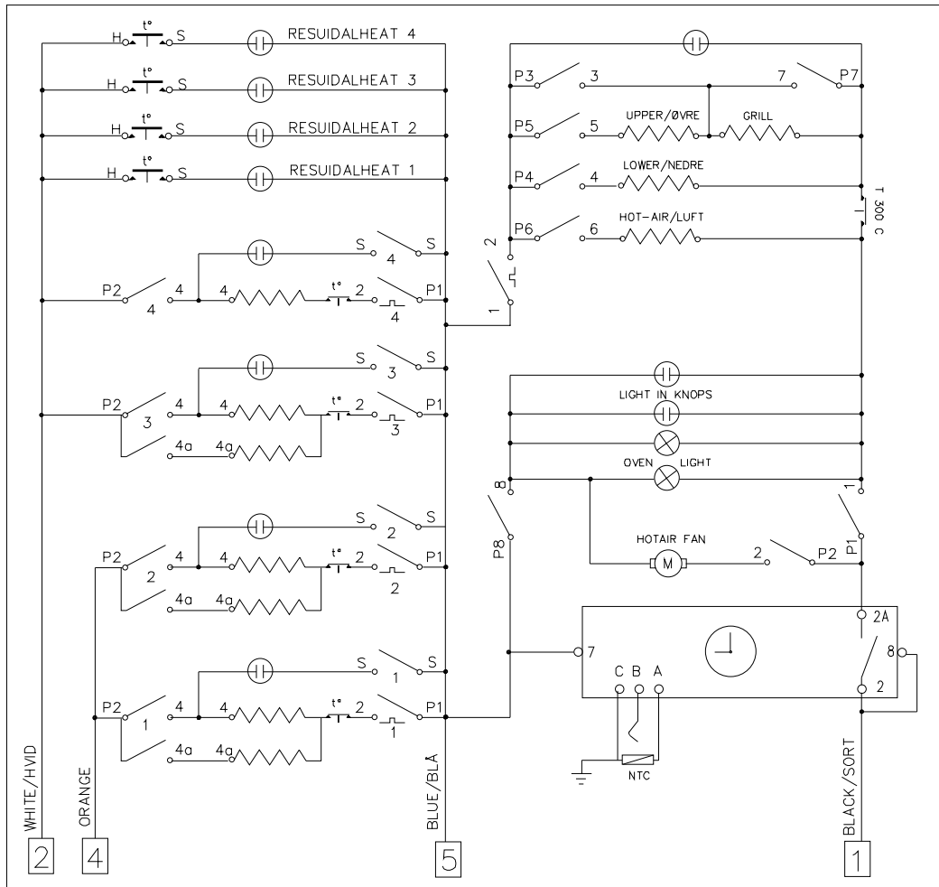
SWITCH F. HOTAIR OVEN/ AFBRYDER F. LUFTOVN
