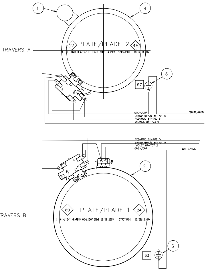
FRONT SET FRA BUNDEN FRONT SEEN FROM BOTTOM WIRINGSET/LEDNINGSSÆT: 80 24 81 REV 4
