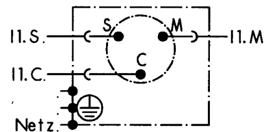
m1 Verdichter-Motor
