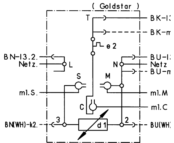
11 Anschlusssteil
