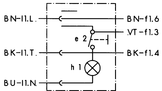
13 Steckbuchse
